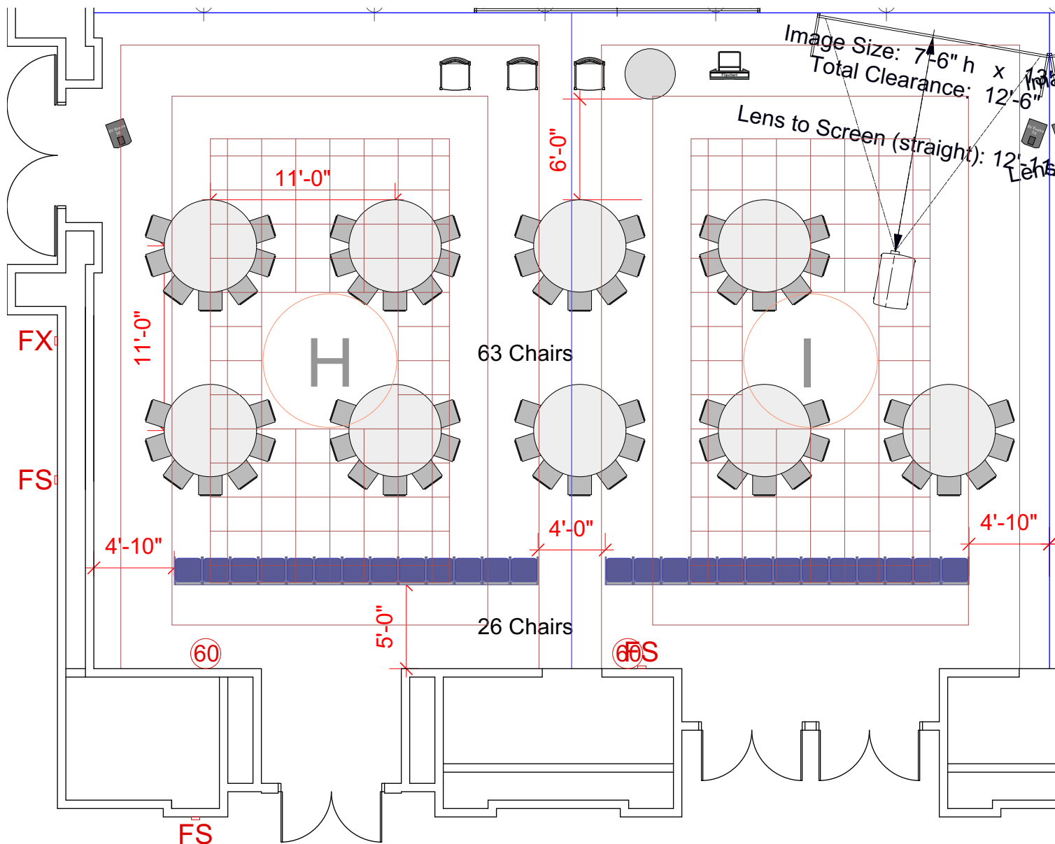
Grand Sonoran HI Scale: 1/8" = 1'-0"
